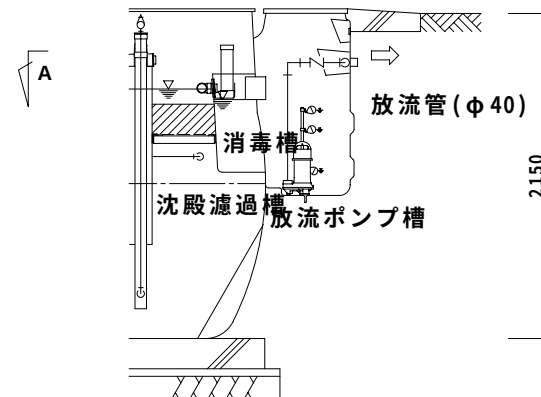
B - B 断面図
