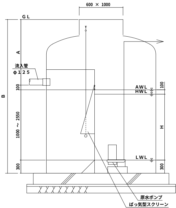
断面図
