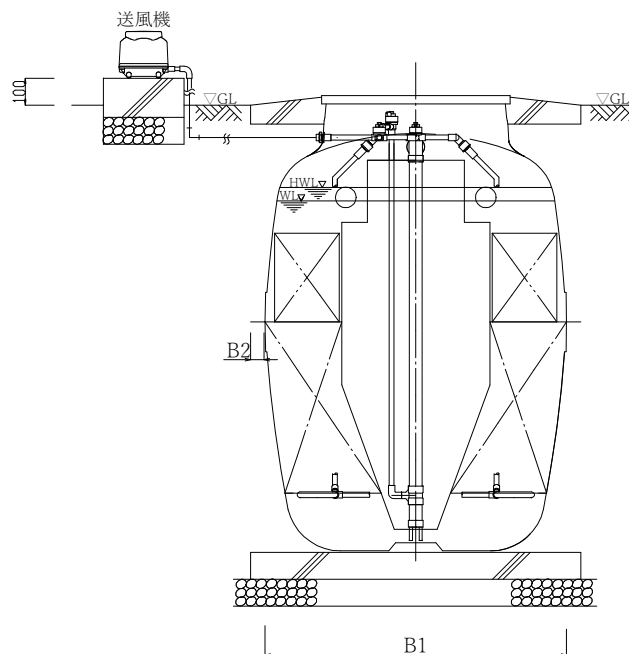
C—C断面図
