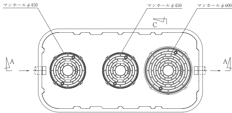
平面图
